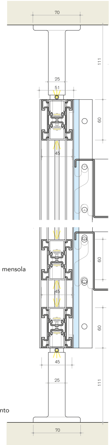
A. particolare a soffitto ceiling detail
