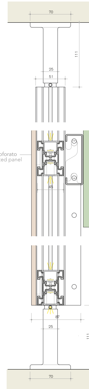
C. particolare a pavimento floor detail
