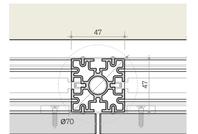
C. sezione orizzontale horizontal section
